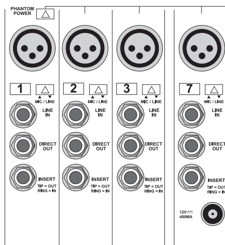
Figura 7.5: Sección de entrada de los canales A y B
