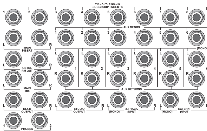
Figura 7.3: Aux Sends, Aux Returns estéreo, Subgrupos Inserts, Más posibilidades de conexión, etc.
