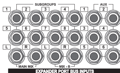
Figura 7.1: Entradas Expander Port
