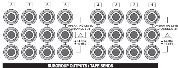
Figura 7.7: Salidas de los subgrupos/Tape Sends y conmutador del nivel de trabajo
